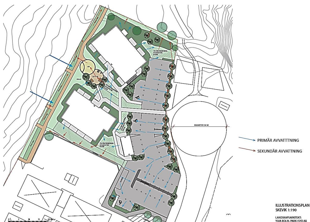
Figur 29 Blå pilar markerar primär avvattning, röda pilar sekundär avvattning.
